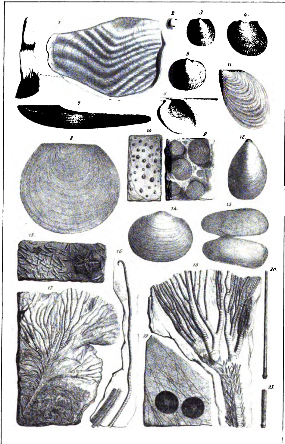
Quenstedt, Jura.
